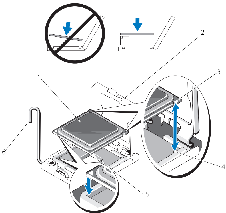
図 3-20. プロセッサの取り付けと取り外し
