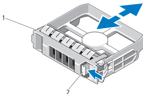
図 3-5. ハードディスクドライブダミーの取り外しと取り付け
