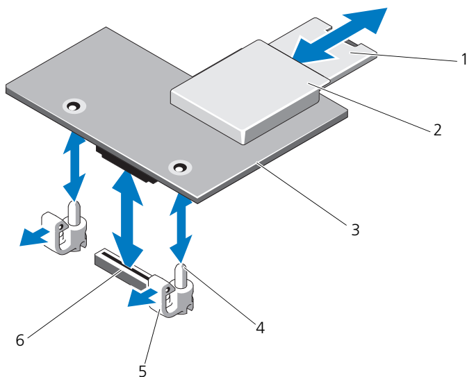
図 3-17. iDRAC6 Enterprise カードの取り付けまたは取り外し
