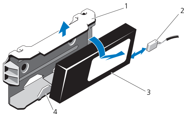
図 3-22. RAID バッテリの取り付けと取り外し
