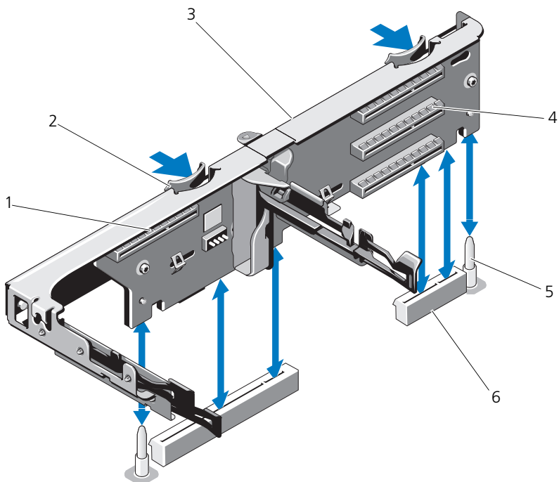
図 3-14. 拡張カードライザーの取り付けまたは取り外し
