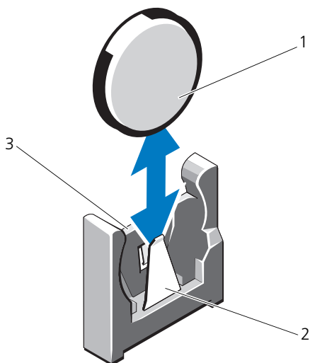
図 3-21. システムバッテリーの交換
