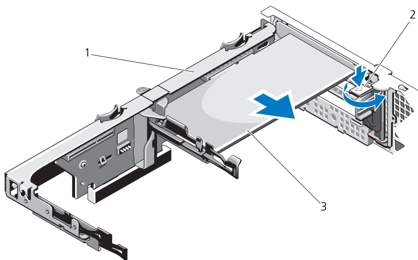
図 3-13. 拡張カードの取り付けまたは取り外し
