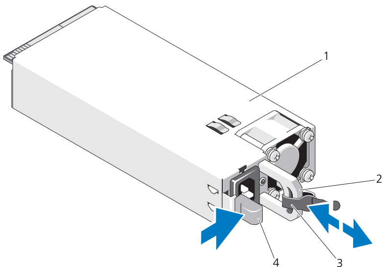
図 3-11. 冗長電源ユニットの取り外しと取り付け
