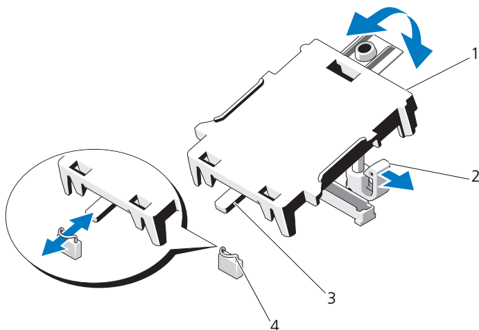
図 3-16. iDRAC6 Express カードの取り付けまたは取り外し
