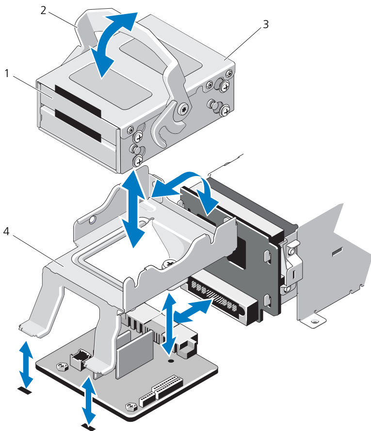
図 3-8. 内蔵ハードディスクドライブベイの取り付けと取り外し
