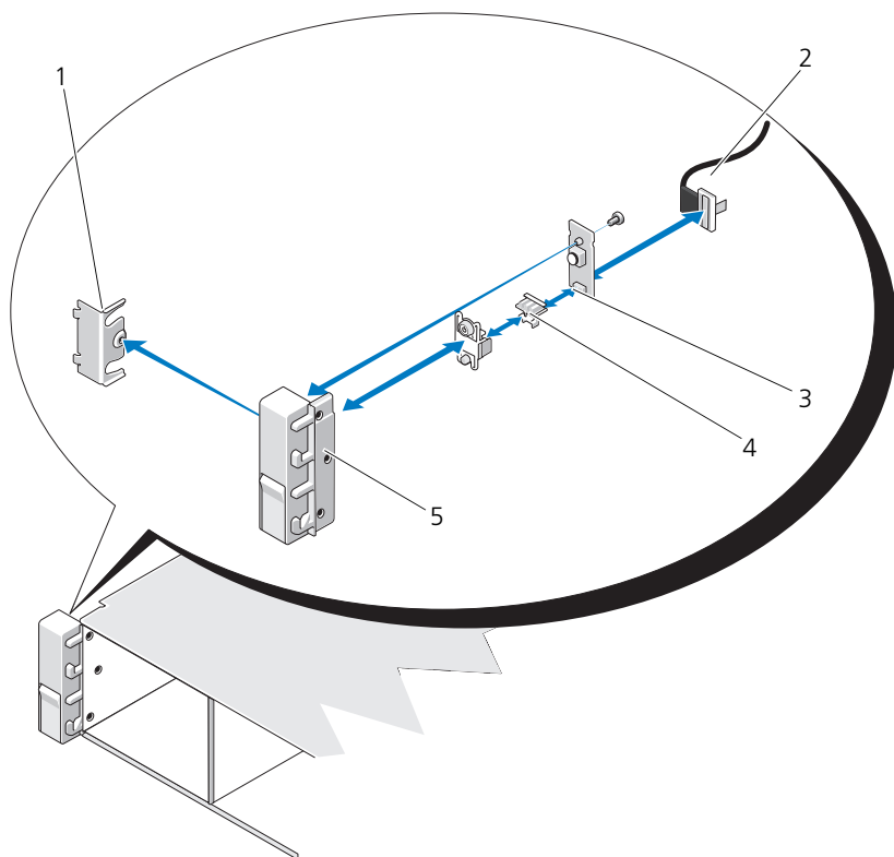
図 3-23. コントロールパネルの取り外しと取り付け
