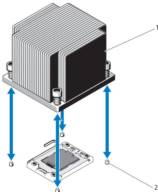
図 3-19. ヒートシンクの取り付けと取り外し
